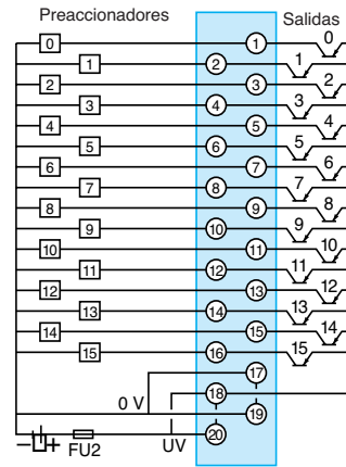
UV: ~ 24 V para TSX DSY 16T2 ~ 48 V para TSX DSY 16T3 FU2: fusible rápido 6,3 A para TSX DSY 16T2 10 A para TSX DSY 16T3
