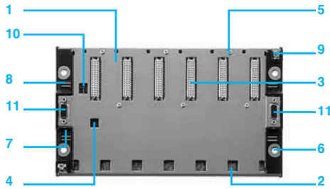
Rack de dirección n (con formato estándar de alimentación) "menos significativo" "más significativo"
