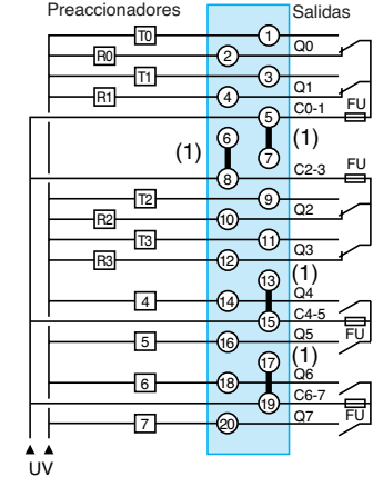
UV: ~ 19...240 V o ~ 19...60 V para TSX DSY 08R5A ~ 24...130 V para TSX DSY 08R4D FU: fusible rápido de 6,3 A (1) La conexión debe realizarse para una fuente de alimentación de ~ 24 V o ~ 24 V
